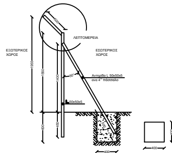
ΠΛΑΓΙΑ ΟΨΗ ΠΑΣΣΑΛΟΥ ΜΕ ΑΝΤΗΡΙΔΑ
